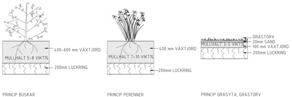
Illustration; Planteringsprincip växtbädd buskar/perenner/gräs
