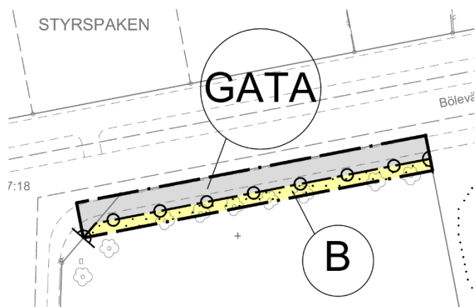
Figur 6: Utdrag ur plankartan för del av fastigheten Aspgården 19. Inom prickmarkerat område får byggnad inte uppföras. Illustration ej i skala.
