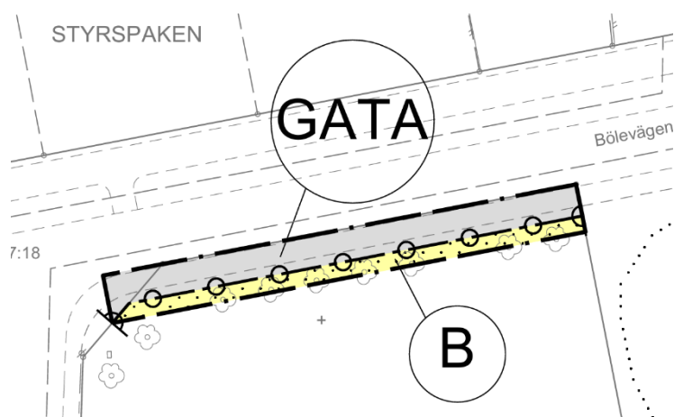
Figur 8: Utdrag ur plankartan, för del av fastigheten Aspgården 19, som visar utfartsförbud (svarta cirklar) mellan allmän platsmark (GATA) och kvartersmark (B). Illustration ej i skala.
