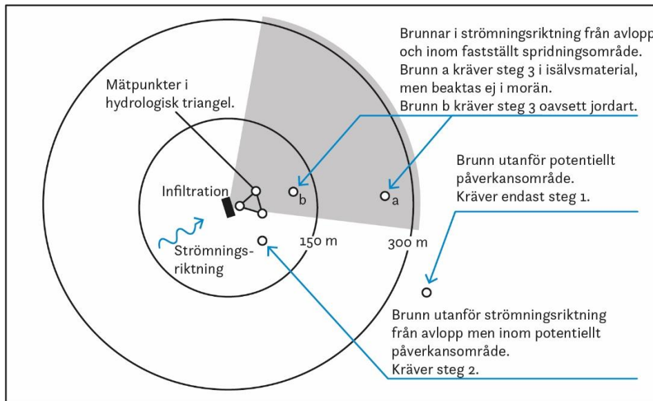
Figur 2. Principskiss över utredningsmodell med exempel på brunnspositioner. Figuren illustrerar gränser för potentiellt påverkansområde i morän (den lilla cirkeln) och isälvsmaterial (den stora cirkeln) samt fastställt spridningsområde (det grå fältet). Vinkeln på det grå fältet kan variera. Med en flackare terräng och därmed svag gradient på grundvattnets lutning, blir spridningen bredare och spridningsriktningen mer oviss.
